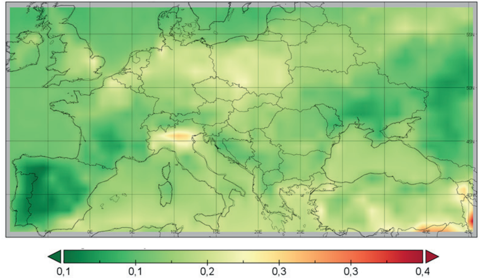
2003-2019 Aerosol Optik Derinliği (AOD) Ortalamaları
